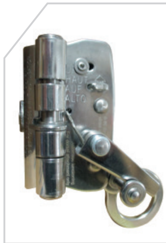
Freno de acero inoxidable con traba para cuerda de 11 a 13 mm. Certificado BUREAU VERITAS N° 301/16-2837.04 Norma: UNE - EN 12841
